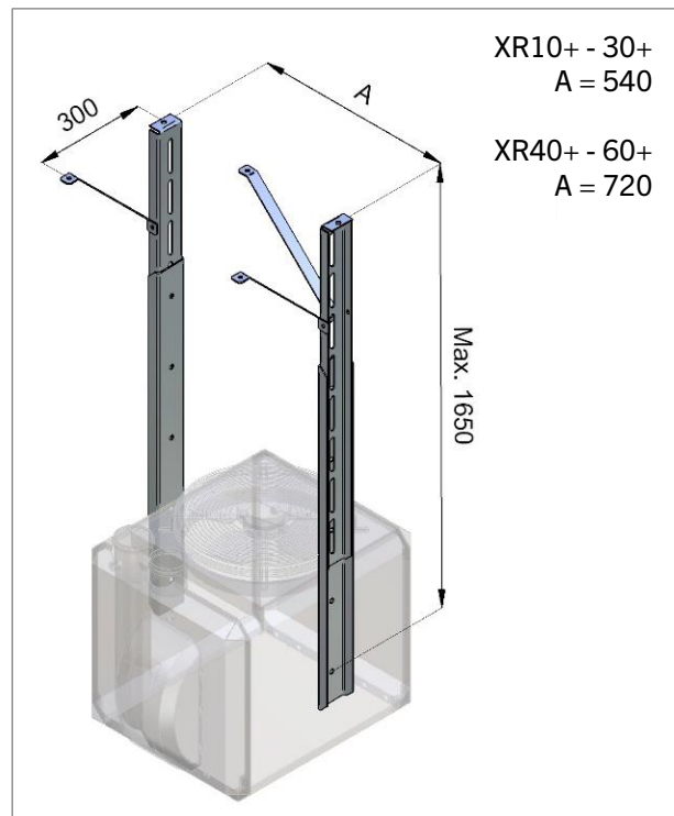
Figuur 6 - Verticale ophangingskit
