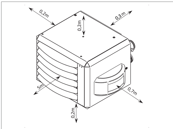
Figuur 3 - Minimale vrije ruimte rondom de luchtverwarmer
