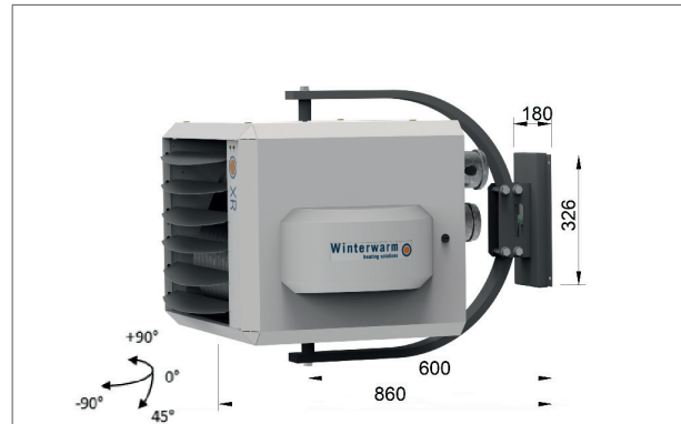
Figuur 5 - Muurconsole (draaibaar)
