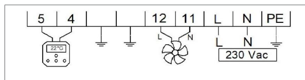
Figuur 7 - De verbindingsklemmen van de luchtverwarmer
