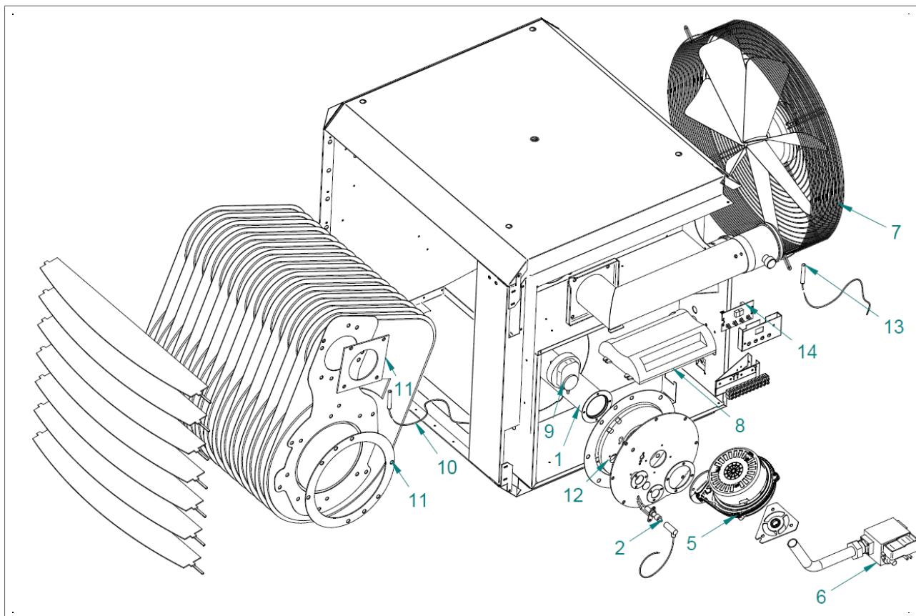
Figuur 24 - Exploded view van de XR10+ - XR60+
