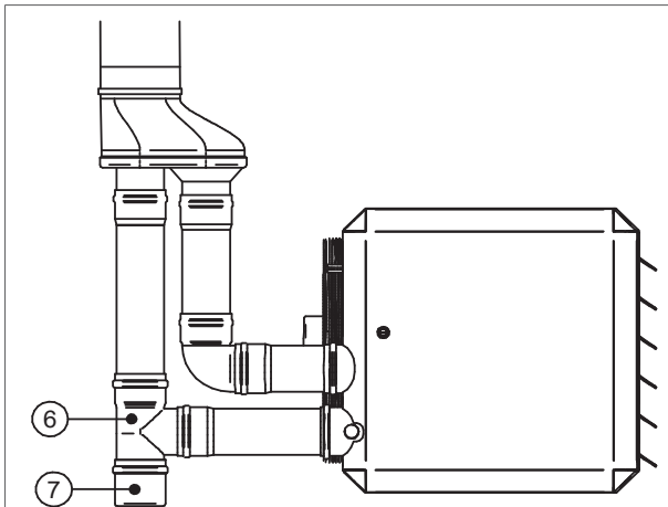
Figuur 14- Een T-stuk (6) en condensaatpot (7)
