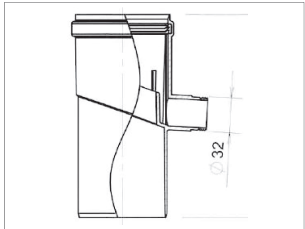
Figuur 15 - Condensaatafvoer
