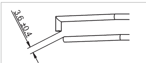
Figuur 21 - Afstand tussen de twee elektroden
