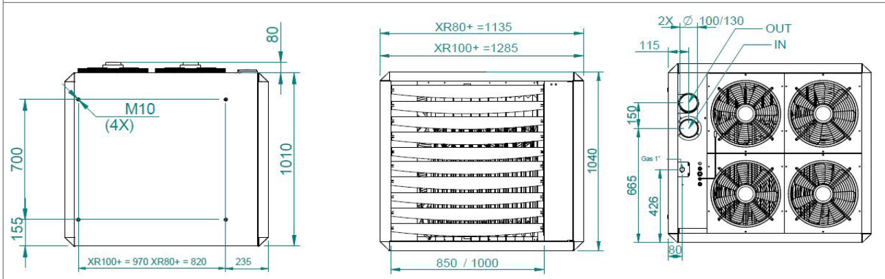
Figuur 2 - Afmetingen van de XR80+ - XR100+
