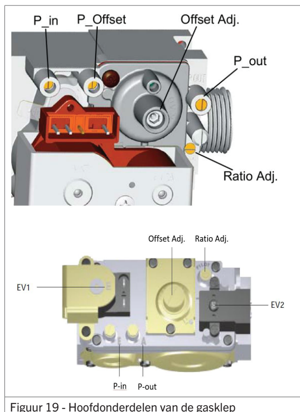
Figuur 19 - Hoofdonderdelen van de gasklep
