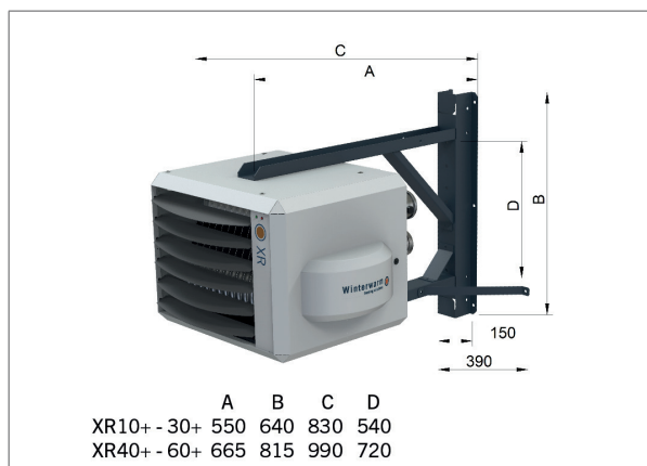
Figuur 4 - Muurconsole (standaard)
