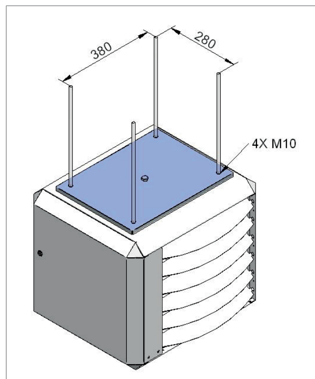
Figuur 7 - Ophangingsadapter
