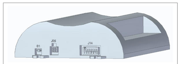
Figuur 11 - Locatie van de S1- en J14-schakelaars
