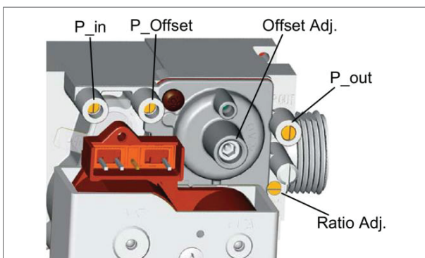
Figuur 22 - Hoofdonderdelen van de gasklep
