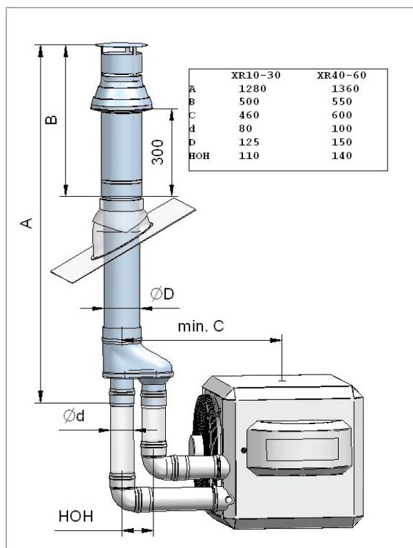
Figuur 15 - Verticale uitmondung XR
