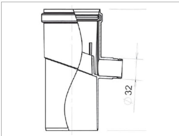
Figuur 18 - Condensaatafvoer
