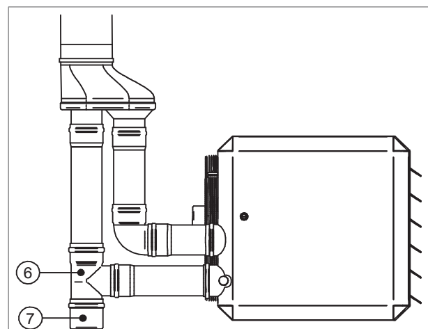
Figuur 17 - Een T-stuk (6) en condensaatpot (7)
