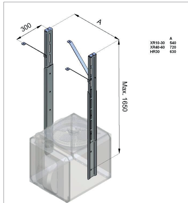
Figuur 6 - Verticale ophangingskit
