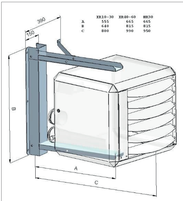
Figuur 4 - Muurconsole (standaard)
