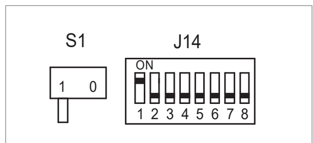
Figuur 10 - Posities van de S1- en J14-schakelaars
