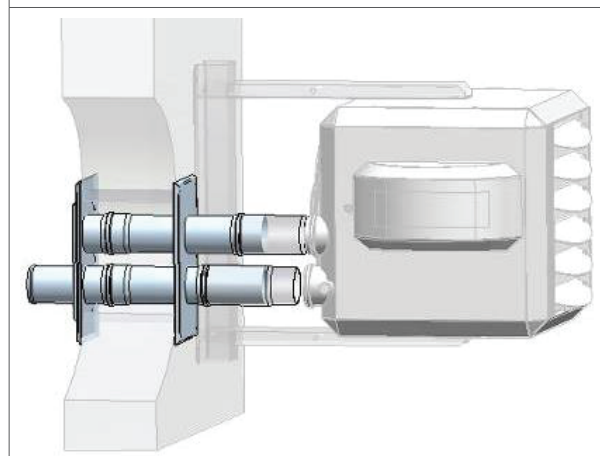
Figuur 16 - Horizontale uitmondung XR
