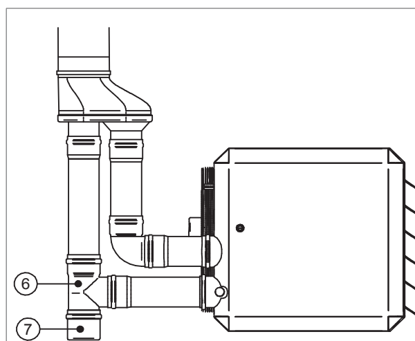
Figuur 13 - Een T-stuk (6) en condensaatpot (7)
